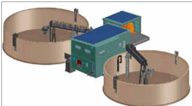
Planungsansicht der zwei neuen SBR-Reaktoren
